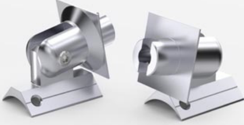
44010 40x40 Hareketli Mafsal Takımı 40x40 Assembled Fitting Set طقم مفصل متحرك 40x40
