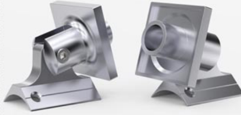
44011 40x40 Hrk. Mafsal Takımı Dışa Geçme 40x40 Assembled Fitting Set Outer Passing طقم مفصل متحرك خارجي 40x40
